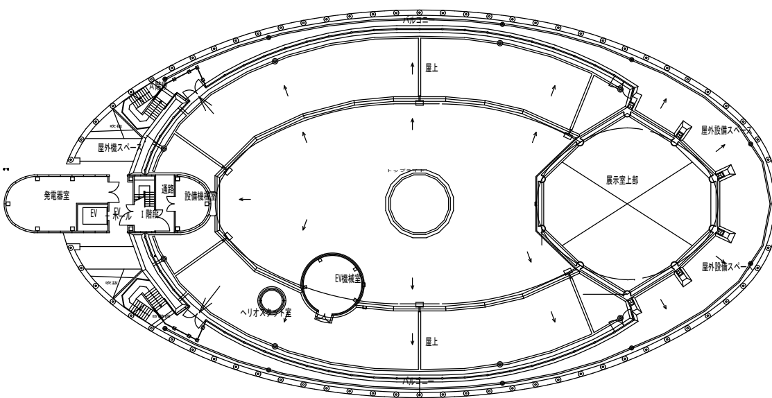
搭屋 1 階
