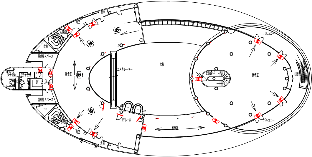
3階
